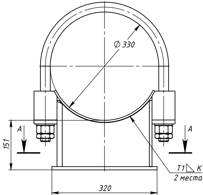
Поз.3 (Ложемент)
