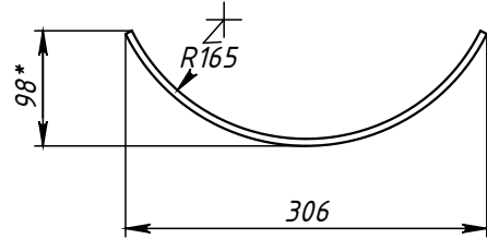
Поз.3 (Ложемент)
