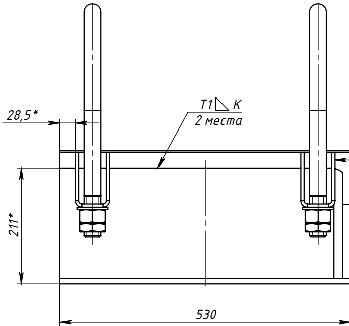
Поз.5 (Хомут)
