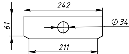
Поз.4 (Ушко) развертка
