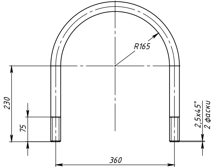
Поз.5 (Хомут)
